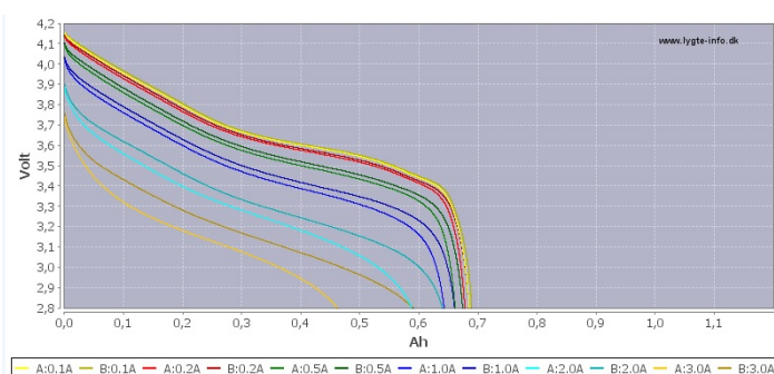
Charakterystyka rozładowania akumulatora XTAR 16340
